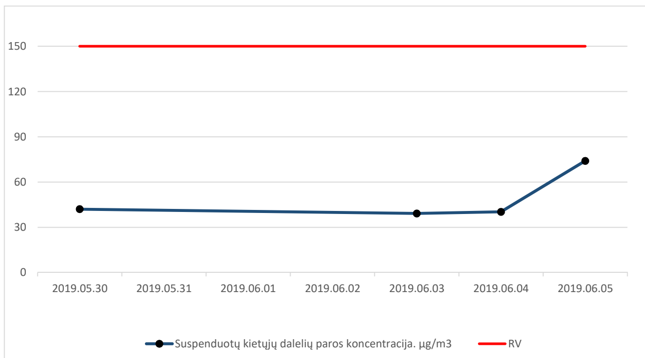
2 pav. Vidutinė paros SKD koncentracija KLASCO teritorijojē N. Uosto g. 23
