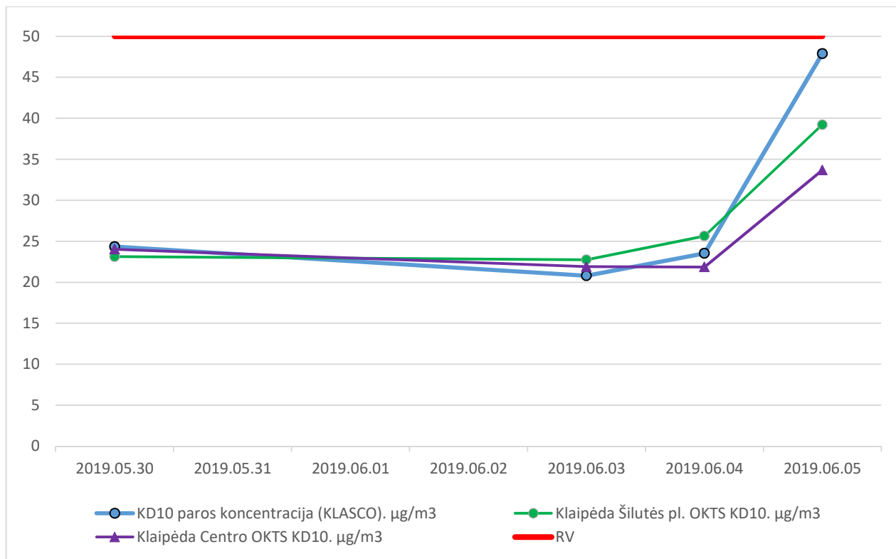
1 pav. Vidutinė paros KD_{10} koncentracija KLASCO teritorijojē N.Uosto g. 23 ir Klaipėdos oro kokybės tyrimų stotyse
